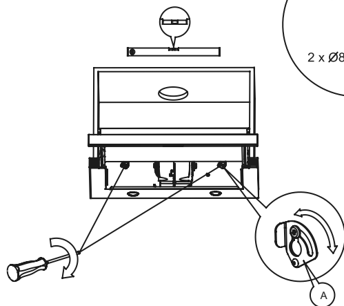
Рис. 6в. Монтаж витяжки
