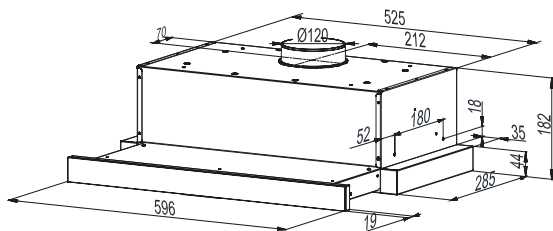
Рис. 2. Габаритні розміри
