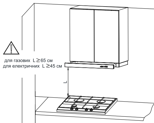
Рис. 2. Рекомендована висота для монтажу витяжки
