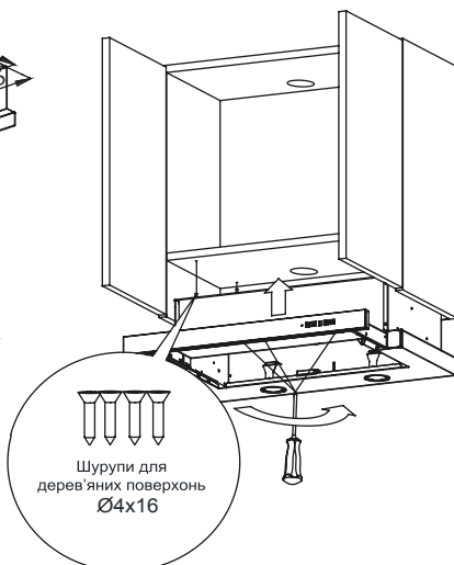
Рис. 5г. Встановлення витяжки – верхнє кріплення
